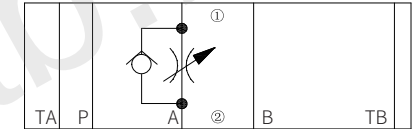
Model Z2FS10A-...-3XJ/...(meter-out control)
