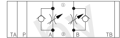
Model Z2FS10-...-3XJ/...(meter-out control)
