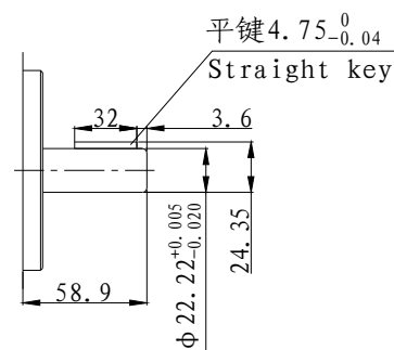
2号轴 (NO SAE) No2. Shaft
