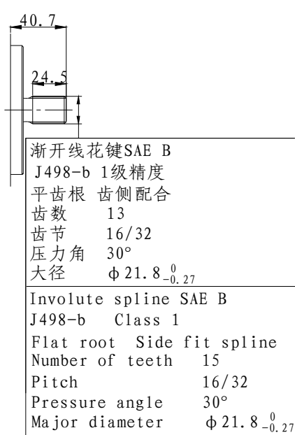
3号轴 No3. Shaft
