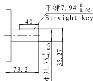
2号轴 (NO SAE) No2. Shaft
