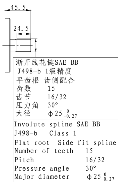
4号轴 No4. Shaft
