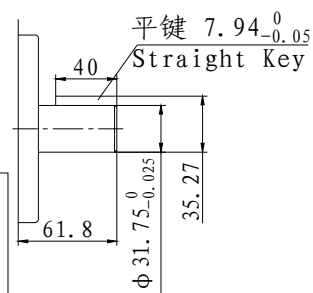
2号轴 (NO SAE) NO. 2 Shaft
