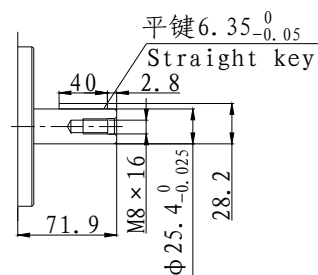
2号轴 (SAE BB) No2. Shaft
