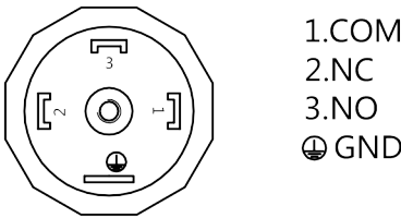
Electrical wiring diagram 电气接线图
