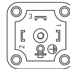
Electrical wiring diagram 电气接线图
