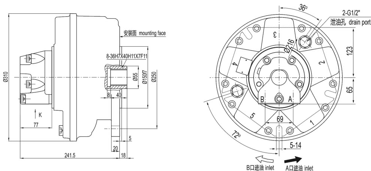
HGM2 外形及安装尺寸/HGM2 Installation Dimensions
