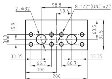
A,C油口/Conn.A,C
