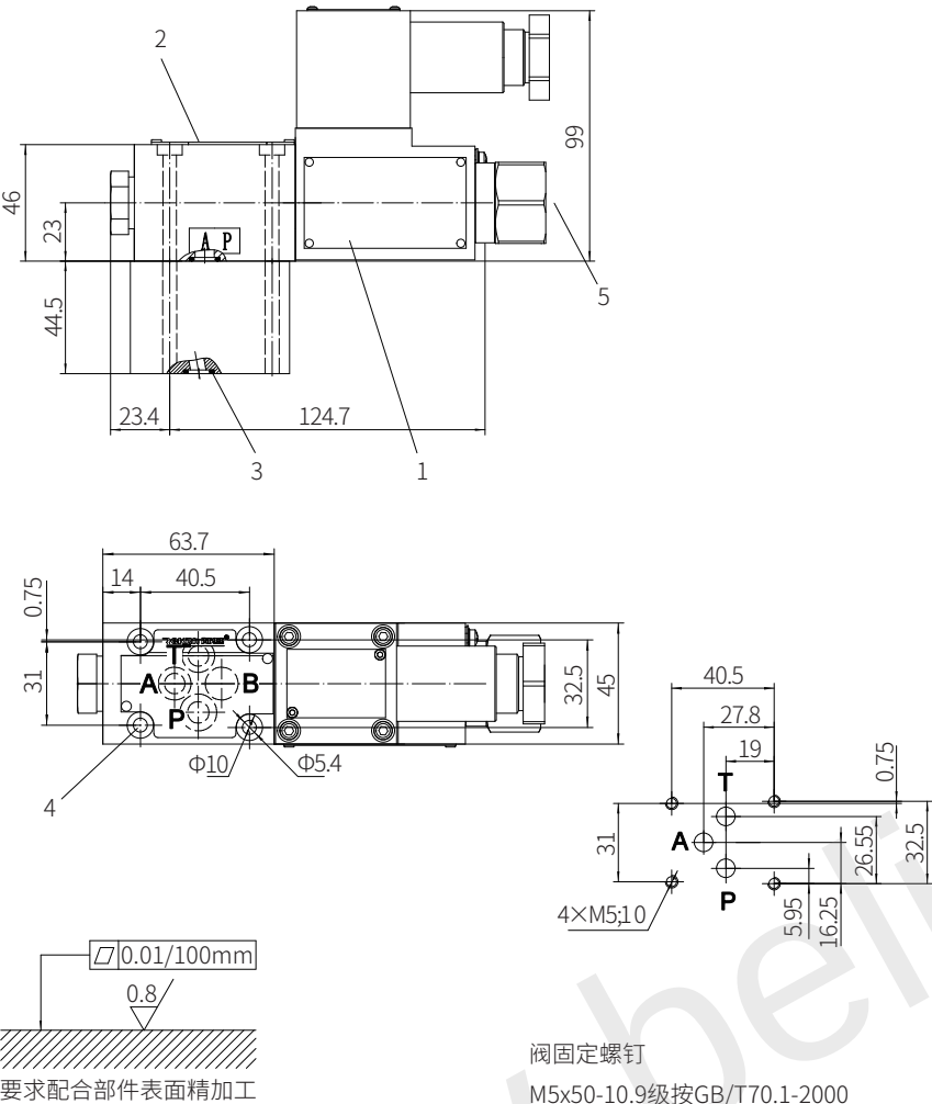
防爆三位四通截止方向阀，“Y”型
